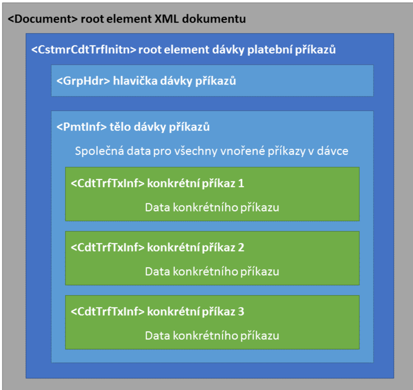
Obr. 1: SCHÉMA ZÁKLADNÍ STRUKTURY XML DOKUMENTU
